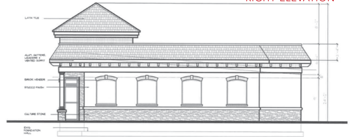
RIGHT ELEVATION
